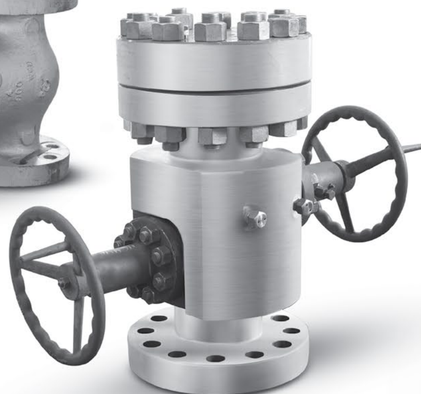
VÁLVULA DOBLE TERMINACIÓN BLOCK DUAL VALVE
